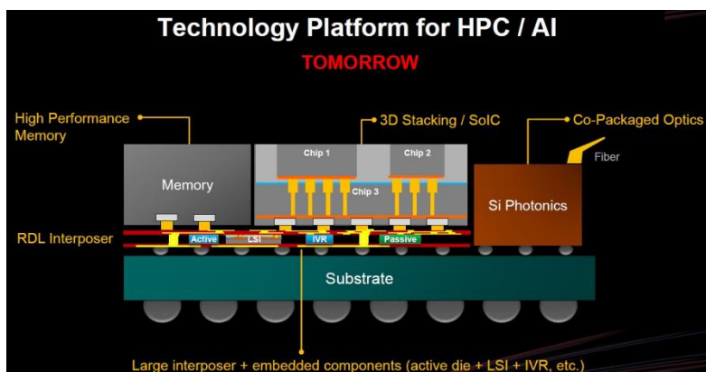
圖二、未來加速器晶片的封裝型態
